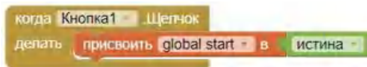
Рисунок 109. Инициализация переменной в обработчике кнопки
