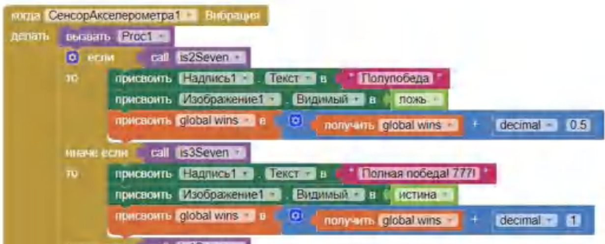
Рисунок 199. Перемена местами блоков is3Seven и is2Seven
