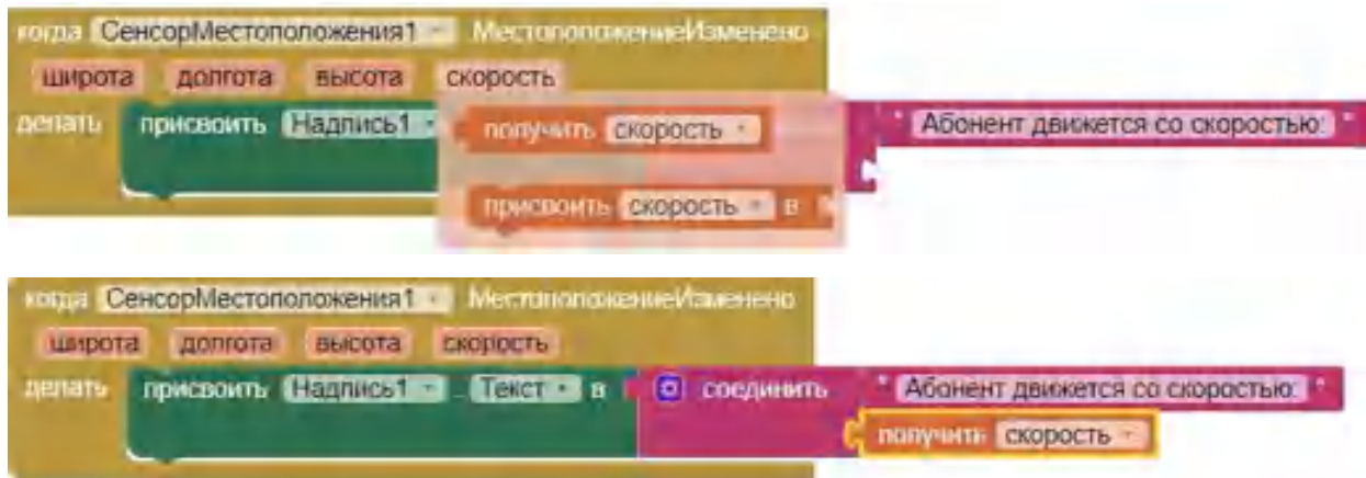
Рисунок 276. Применение внутренней переменной блока
