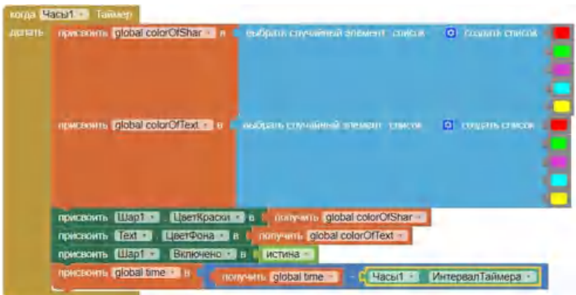
Рисунок 204. Блоки в обработчике событий таймера
