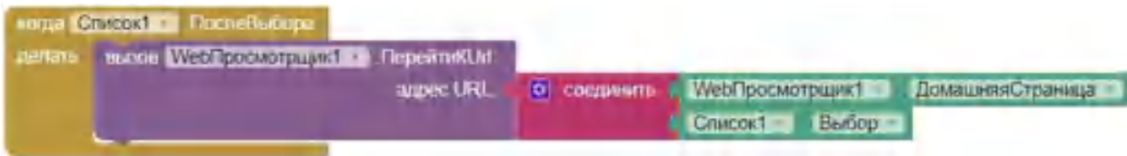
Рисунок 224. Обработка события выбора элемента списка
