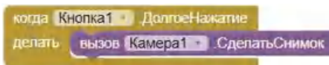
Рисунок 287. Обработчик события «долгое нажатие» на кнопку
