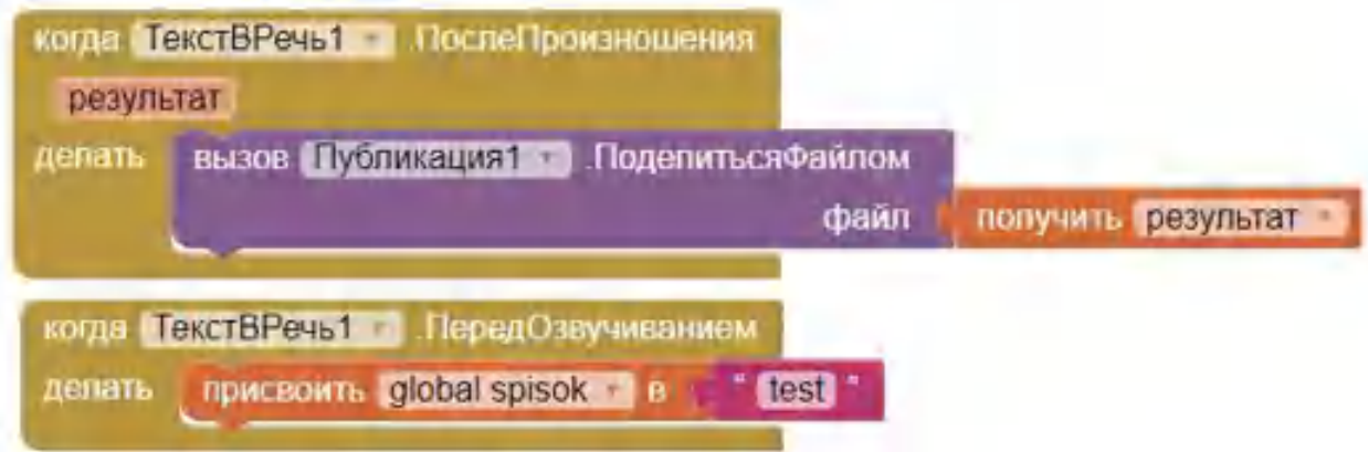
Рисунок 166. Пред- и постобработчики компоненты ТекстВРечь
