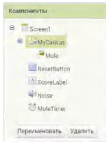
Рисунок 44. Функционал «Компоненты»
