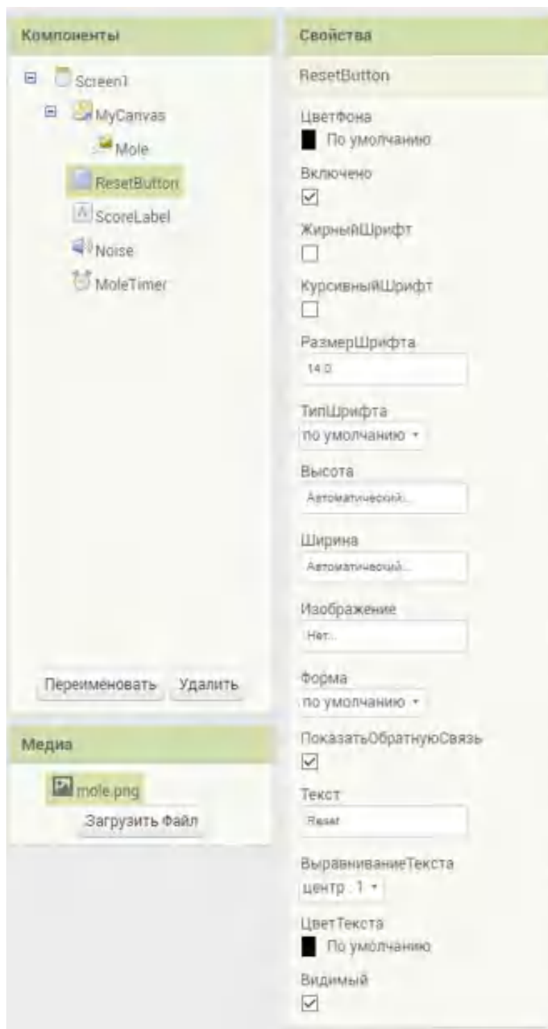
Рисунок 46. Функционал «Свойства»
