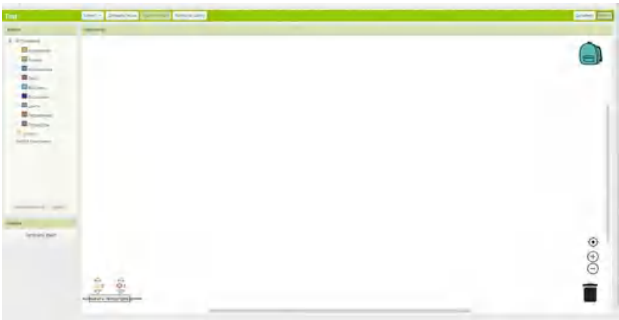
Рисунок 47. Окно «Блоков»
