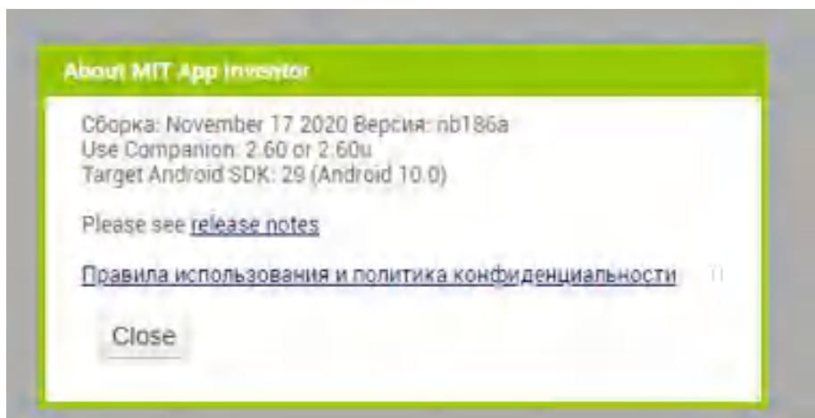
Рисунок 31. Функционал «О»
