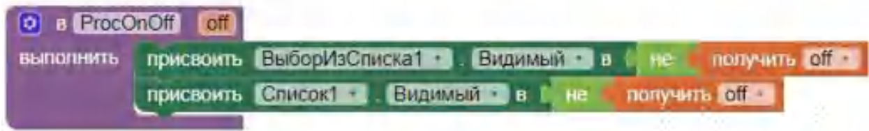
Рисунок 173. Процедура ProcOnOff
