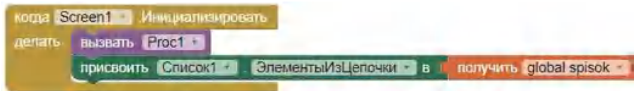
Рисунок 264. Инициализация экрана
