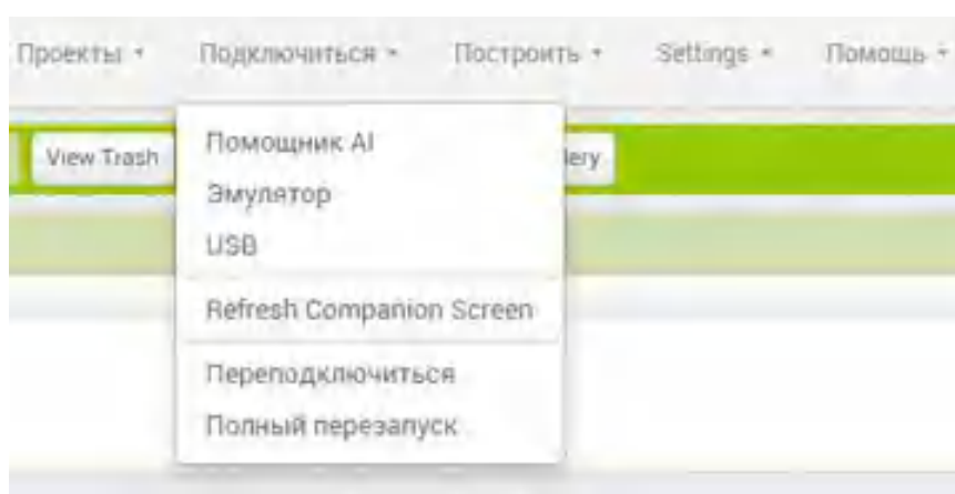
Рисунок 27. Меню «Подключиться»
