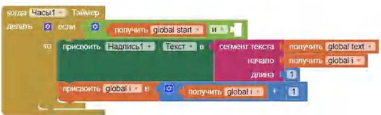
Рисунок 116. Промежуточный вид 3 схемы блоков обработчика таймера
