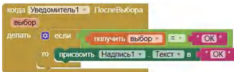
Рисунок 89. Пример обработки ответа пользователя
