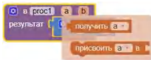
Рисунок 80. Работа с параметрами процедуры
