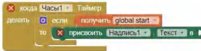
Рисунок 111. Начальная схема блоков обработчика таймера
