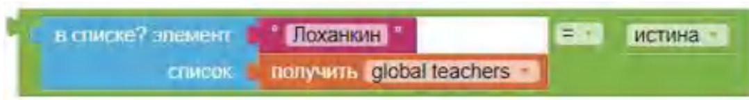
Рисунок 138. Логическое выражение с блоком проверки
