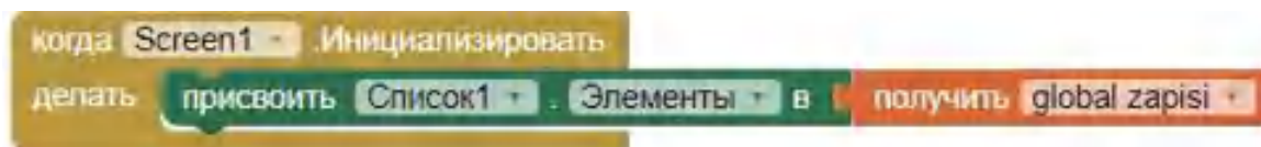
Рисунок 223. Инициализация экрана
