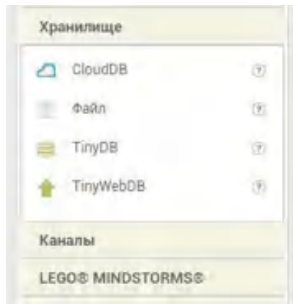
Рисунок 43. Функционал «Хранилище»
