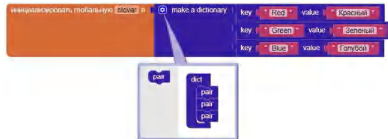
Рисунок 262. Инициализация словаря
