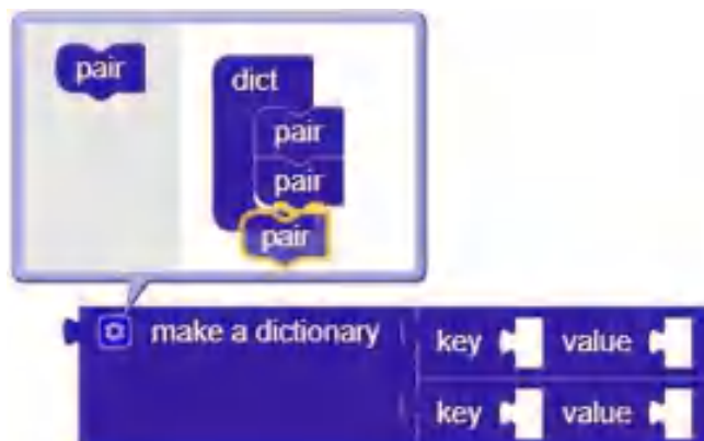
Рисунок 254. Применение мутатора
