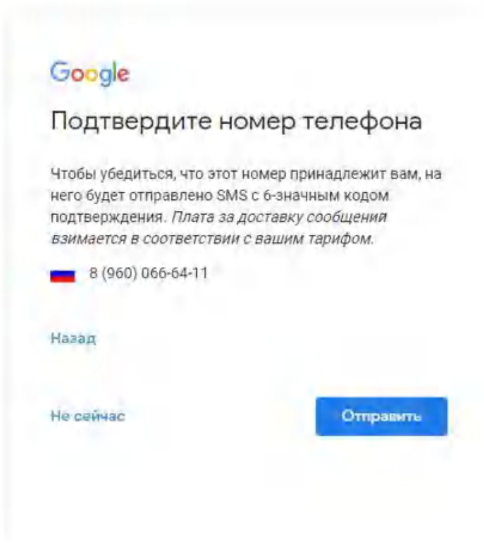
Рисунок 9. Подтверждение номера
