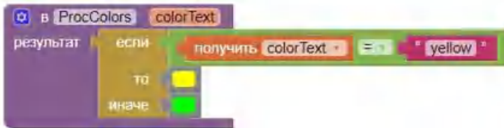
Рисунок 171. Процедура ProcColors
