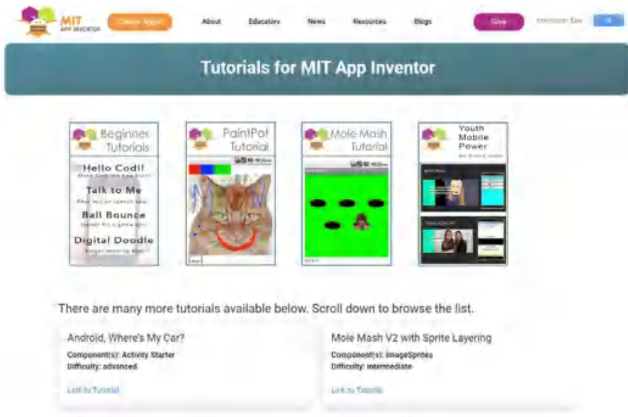
Рисунок 32. Функционал «Уроки»
