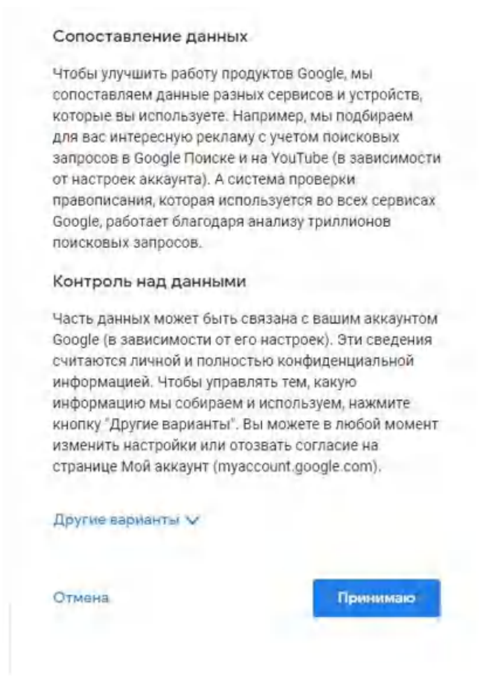
Рисунок 12. Подтверждение договора
