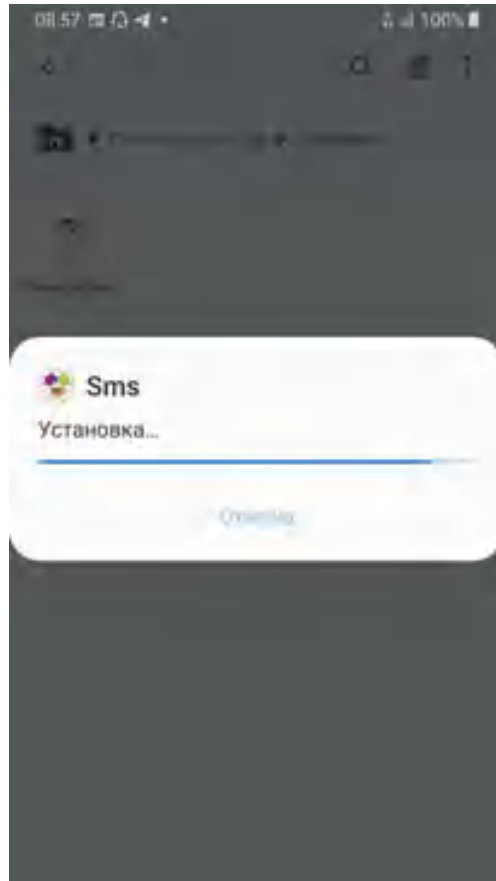
Рисунок 289. Установка приложения
