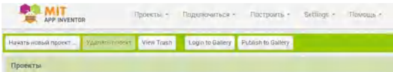
Рисунок 20. Проекты
