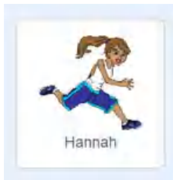
Рис. 196. Вид персонажа
