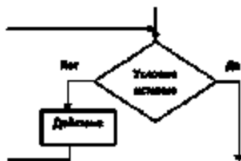
Рис. 109. Блок-схема цикла
