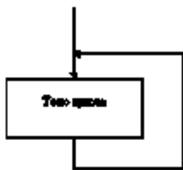
Рис. 108. Блок-схема цикла
